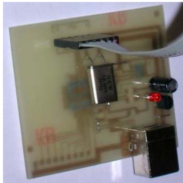
Программатор вид сверху
